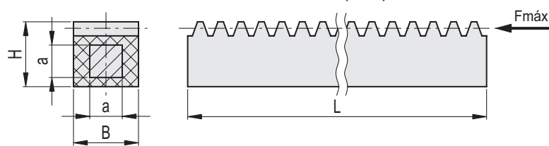
ZCR-A (M ≤ 3)
