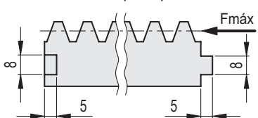
ZCR-A (M = 4)
