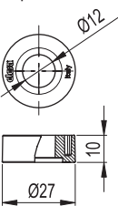
Espaciadores
