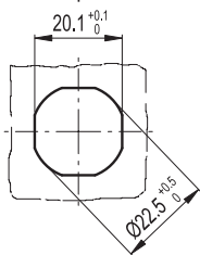
Plantilla de perforación
